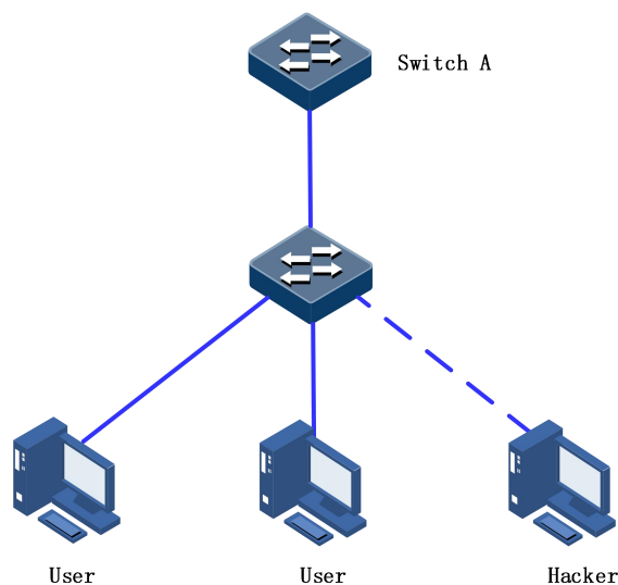
图 1-16 DOS 防攻击应用组网示意图
